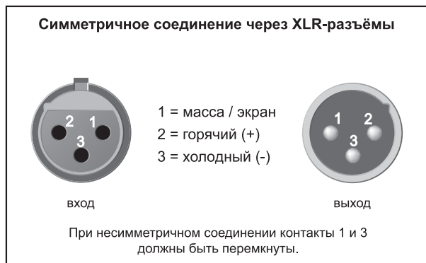
Рис. 4.2: Штекер XLR
