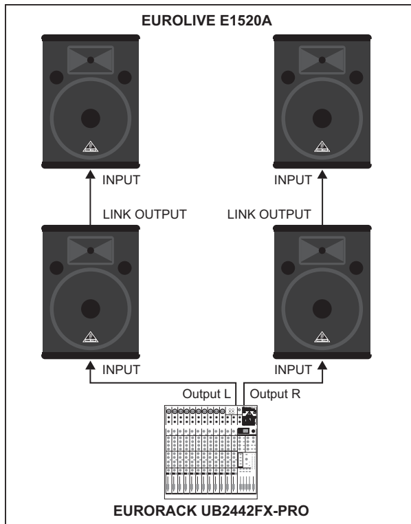
Рис. 3.1: Каскадное соединение нескольких E1220A/E1520A с помощью разъема LINK OUTPUT
