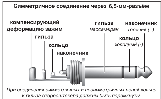
Рис. 4.1: 6,3-миллиметровый стереоштекер
