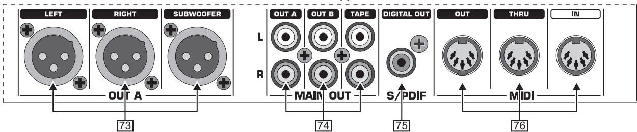
Рис. 2.8: Выходы DDM4000
