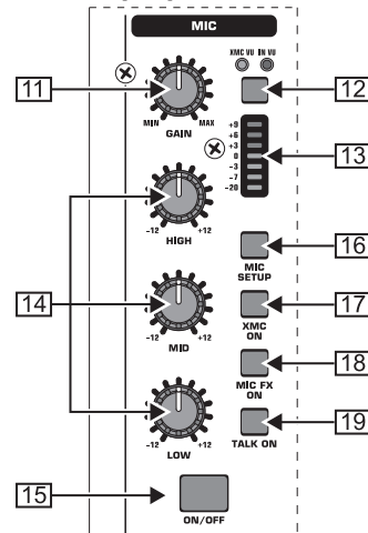
Рис. 2.2: Микрофонный канал
