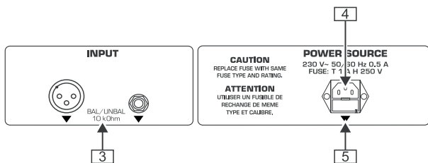
Рис. 2.2: Разъемы на задней панели TRUTH
