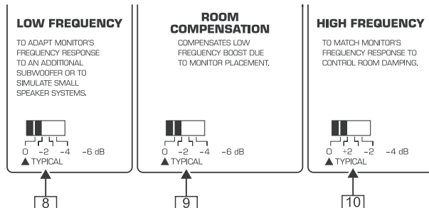
Рис. 2.5: Переключатели на задней панели TRUTH
