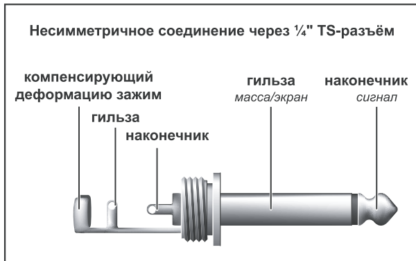
Рис. 4.1: 6,3 мм-моноштекер
