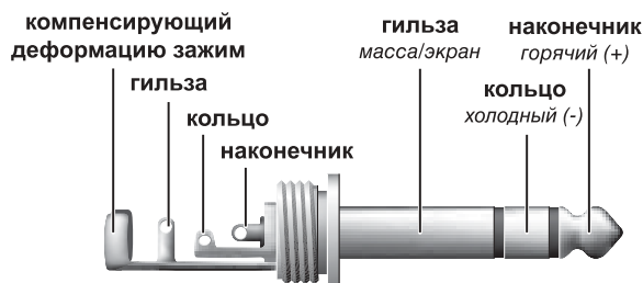
Рис. 4.1: 6,3-миллиметровый стереоштекер
