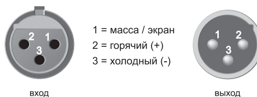
Рис. 4.2: Штекер XLR
